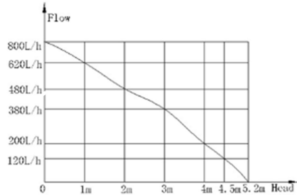
特性曲线图
